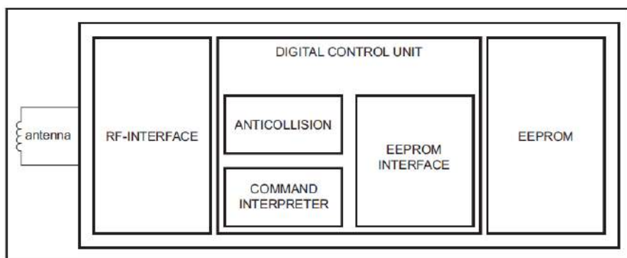
Σχήμα Β1: Διάγραμμα Μπλοκ Ultralight
